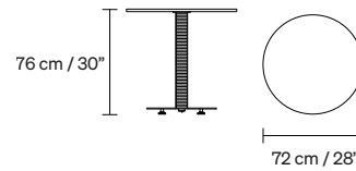
BARCELONETTE ROUND BISTRO TABLE 20.6 kg / 45.5 lb
