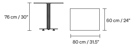
BARCELONETTE RECTANGLE BISTRO TABLE 22.4kg / 49.5 lb
